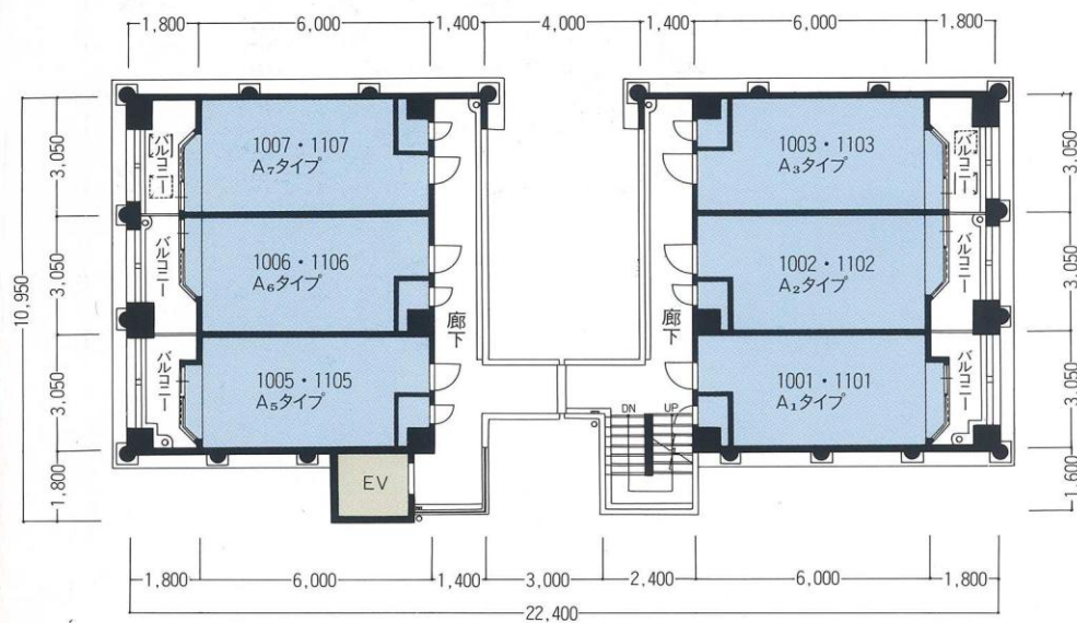
10F・11F平面図
