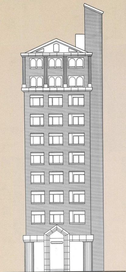
北側立面图
