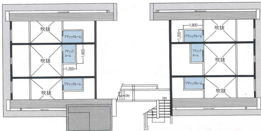
RF平面図
