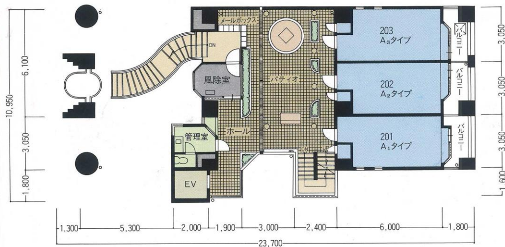
2F平面図
