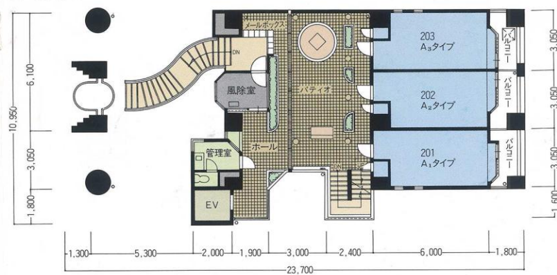
2F平面図
