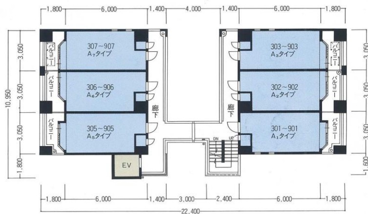
3F～9F平面図
