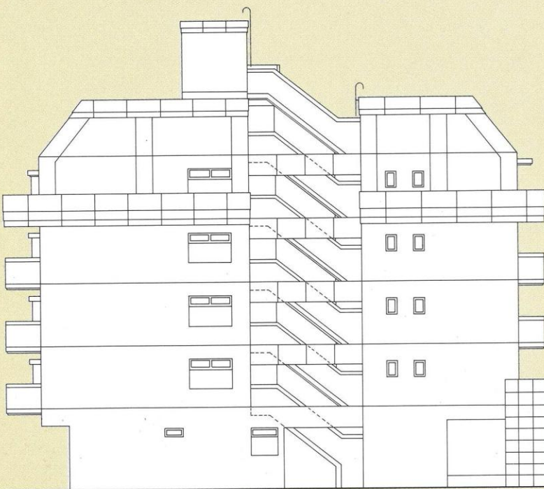
西側立面図
