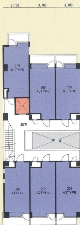
2F 平面図
