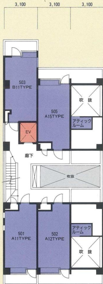
5F 平面図
