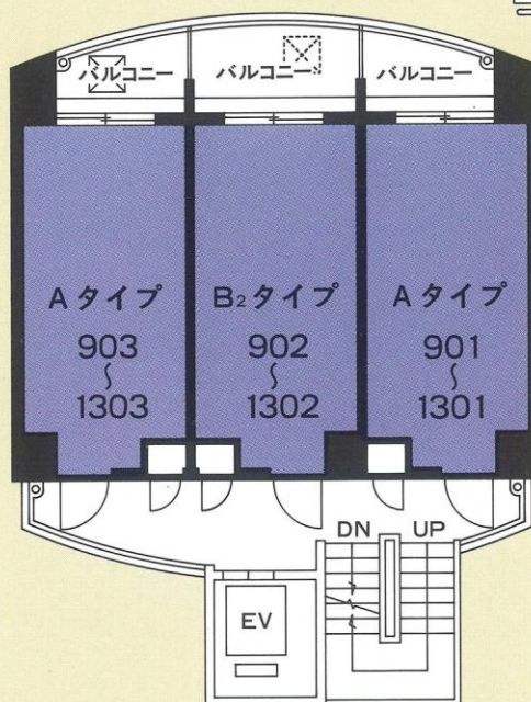
9F~13F平面図
