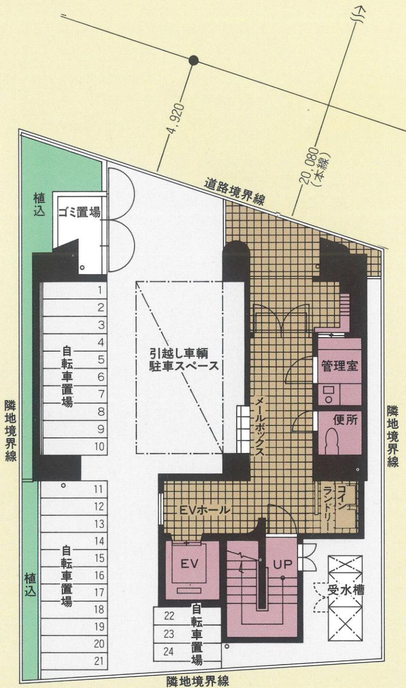
配置図, 1F 平面図
