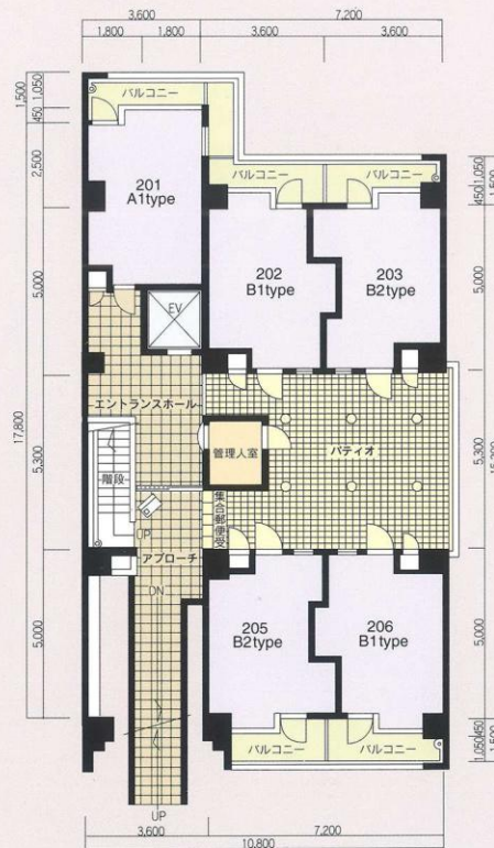
2F平面図
