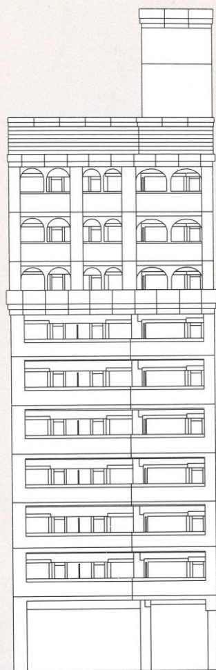
北側立面図
