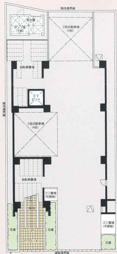
配置図・1F平面図
