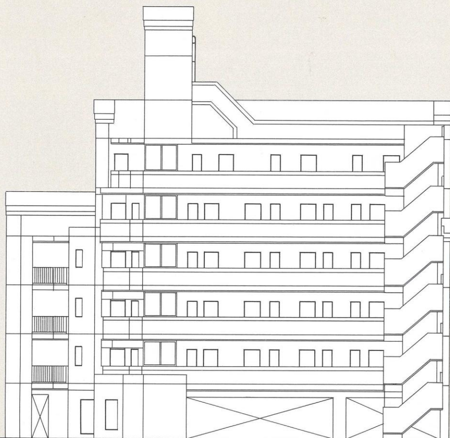
北側立面図
