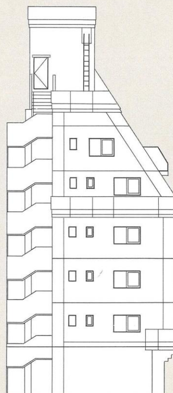
西側立面図
