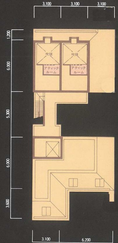
6Fアティック平面図
