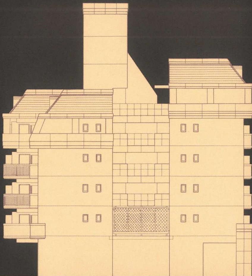
東側立面図
