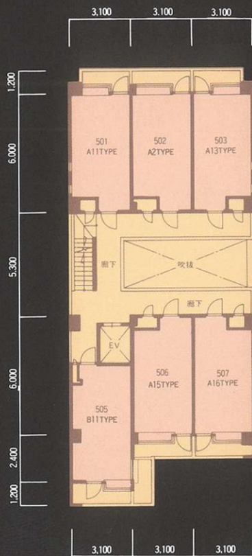
5F平面図
