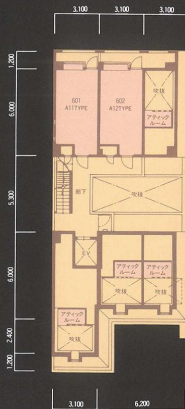
6F平面図
