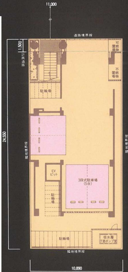
配置図, 1F平面図
