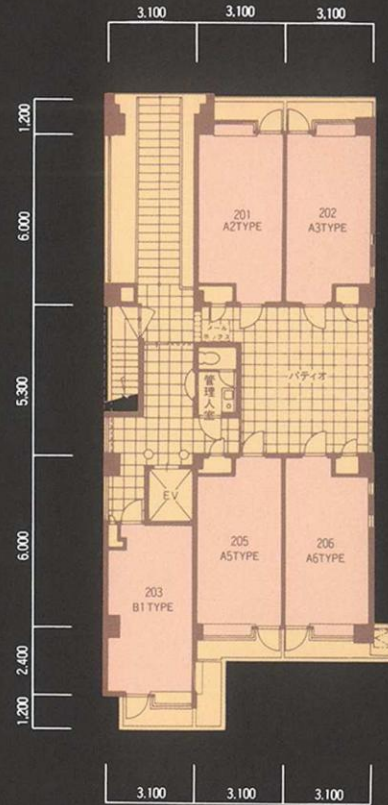
2F平面図
