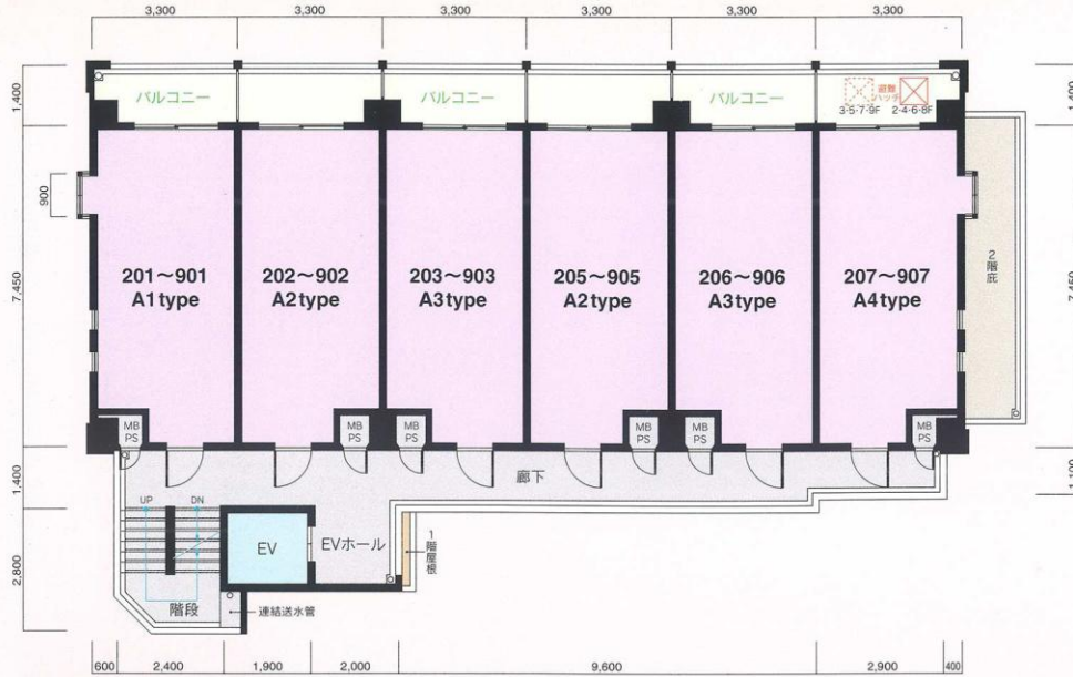
2階～9階平面図
