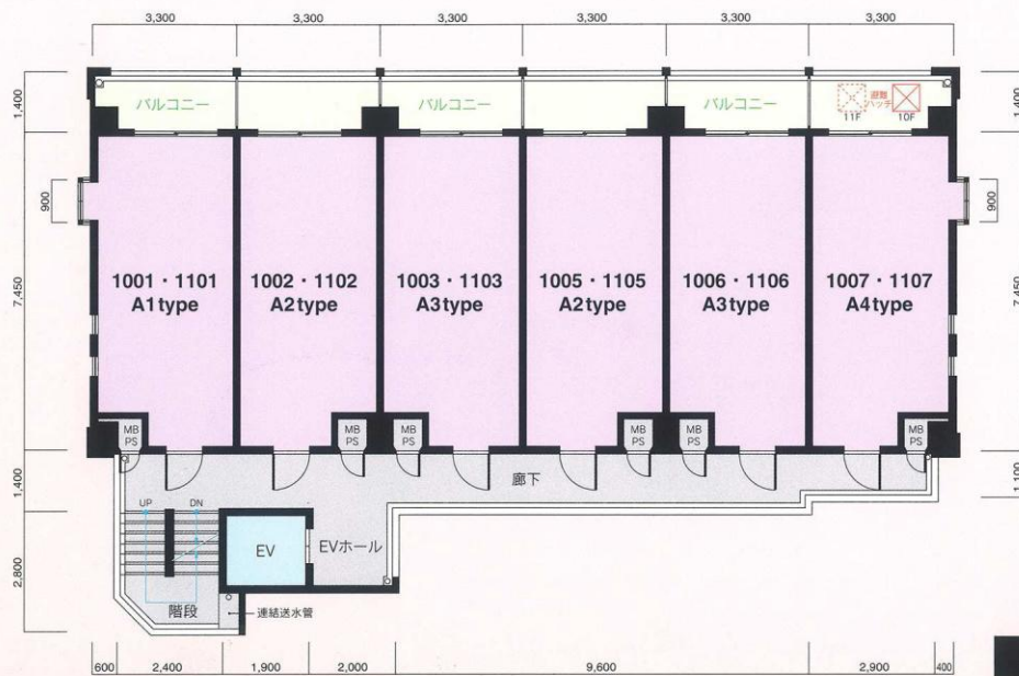
10・11階平面図
