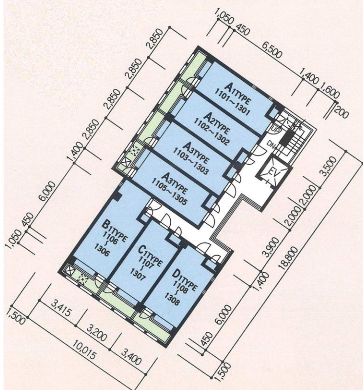
11~13階平面図
