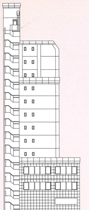
西側立面図
