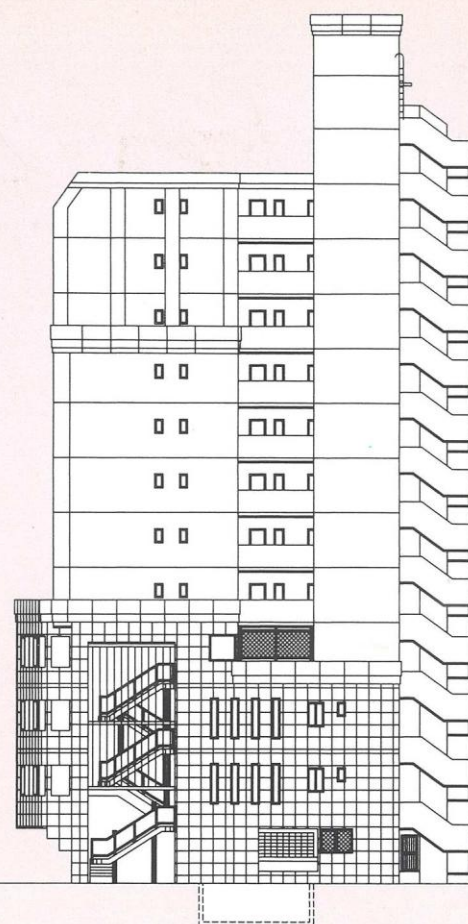
北側立面図
