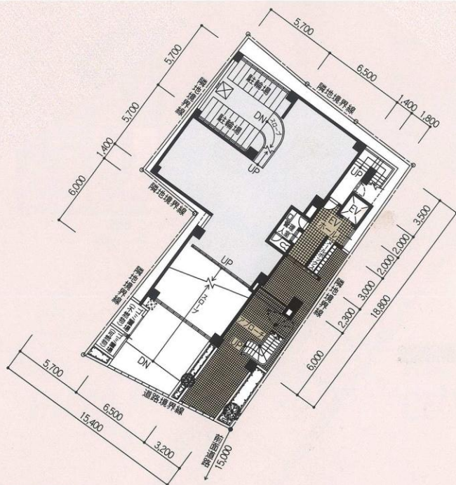
配置図・2階平面図
