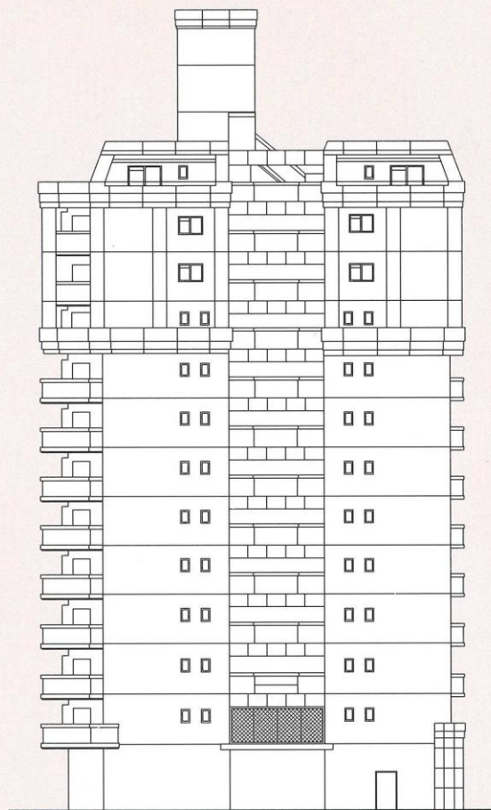
东侧立面图
