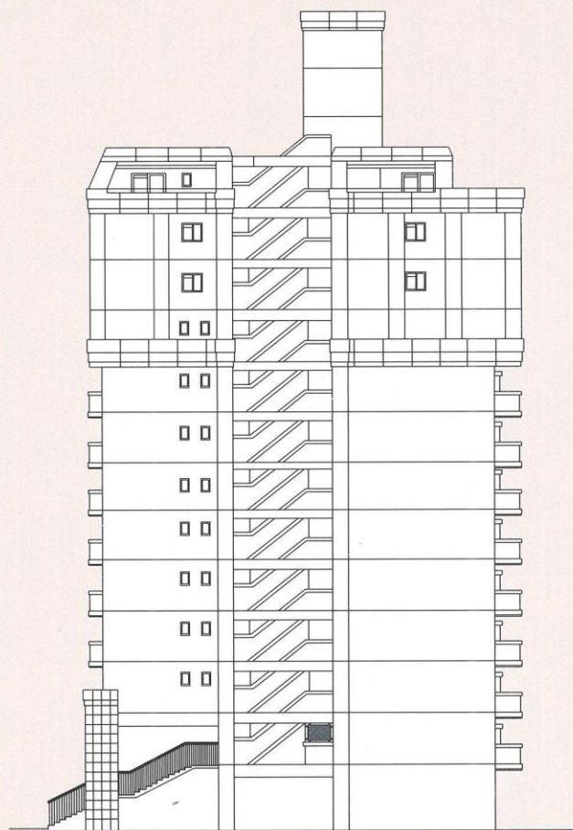
西側立面图
