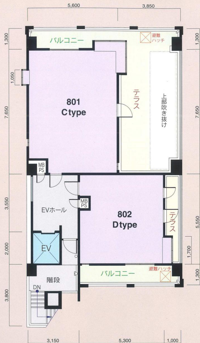
8階平面図
