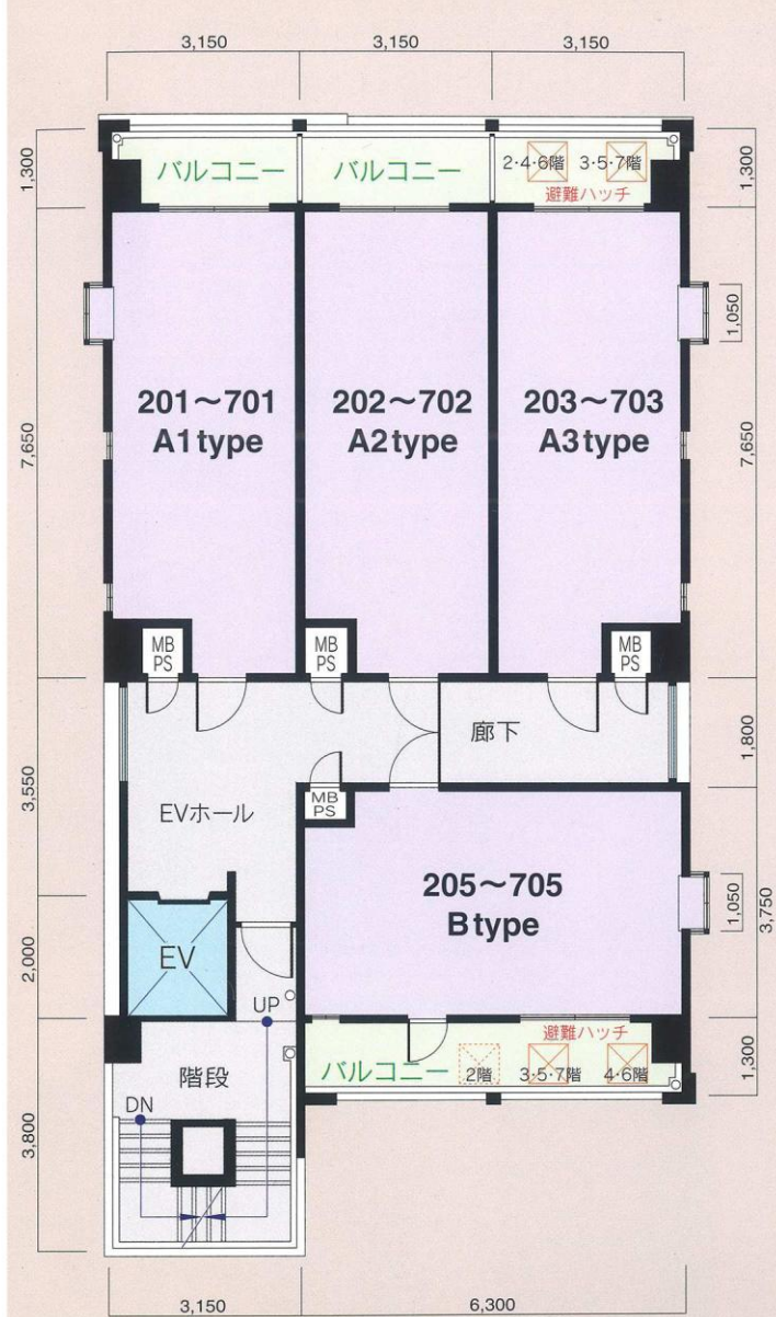
2階～7階平面図
