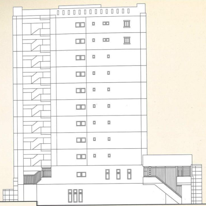
北侧立面图
