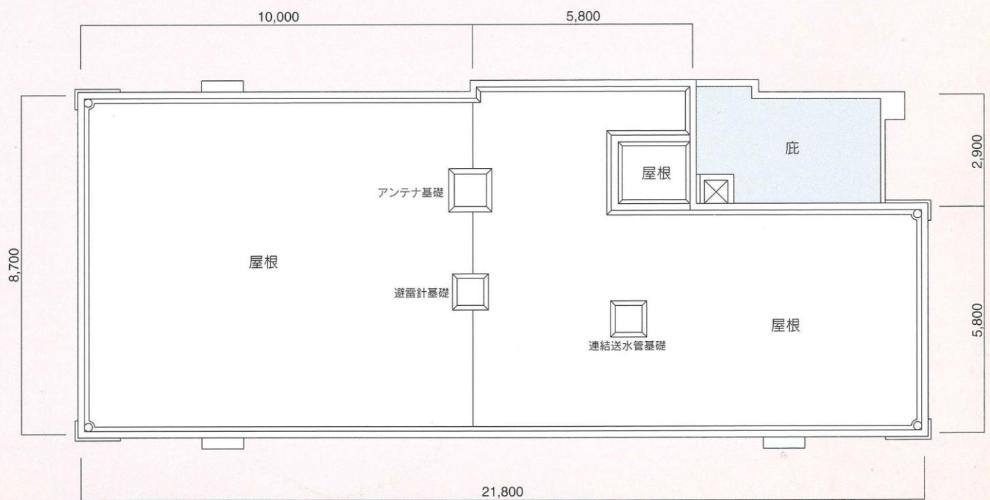
R階平面図
