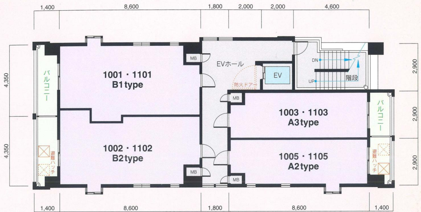
10・11階平面図
