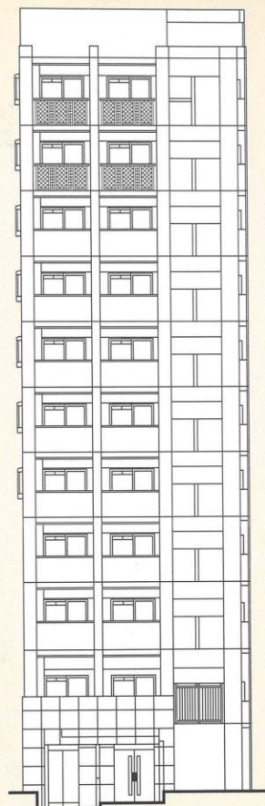
東側立面图
