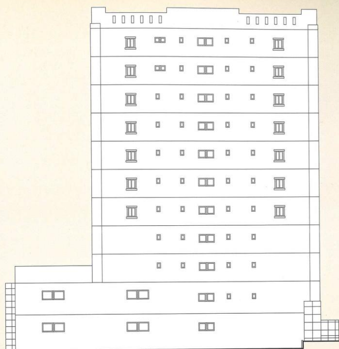
南侧立面图
