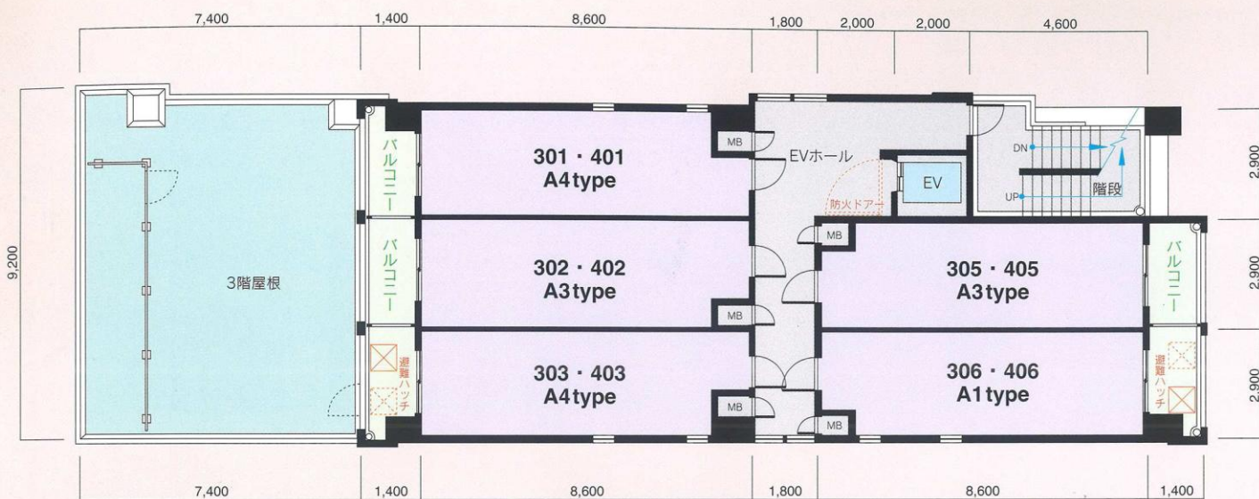
3・4階平面図
