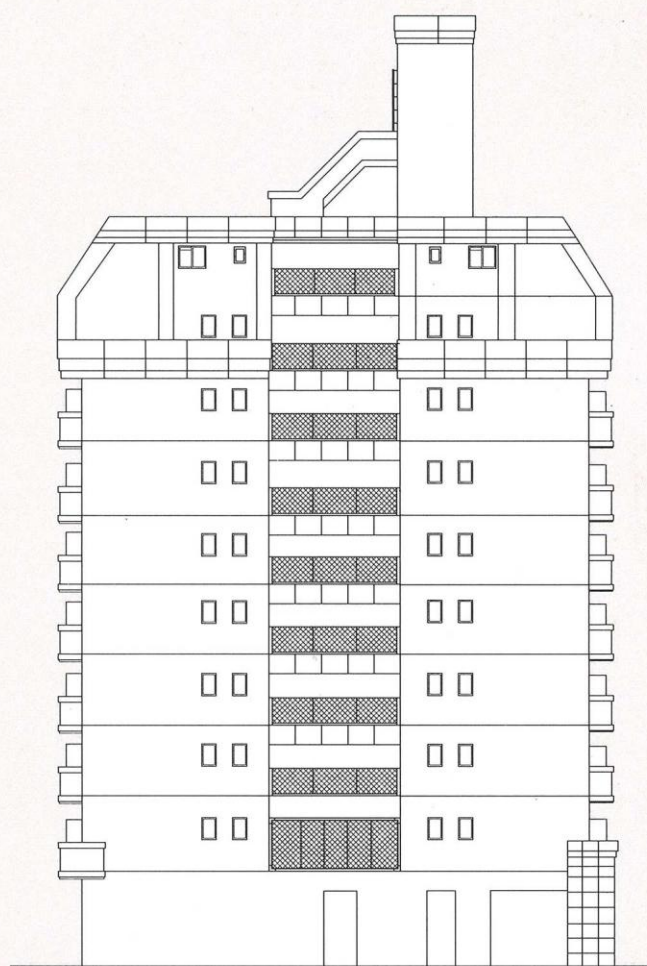
東側立面图
