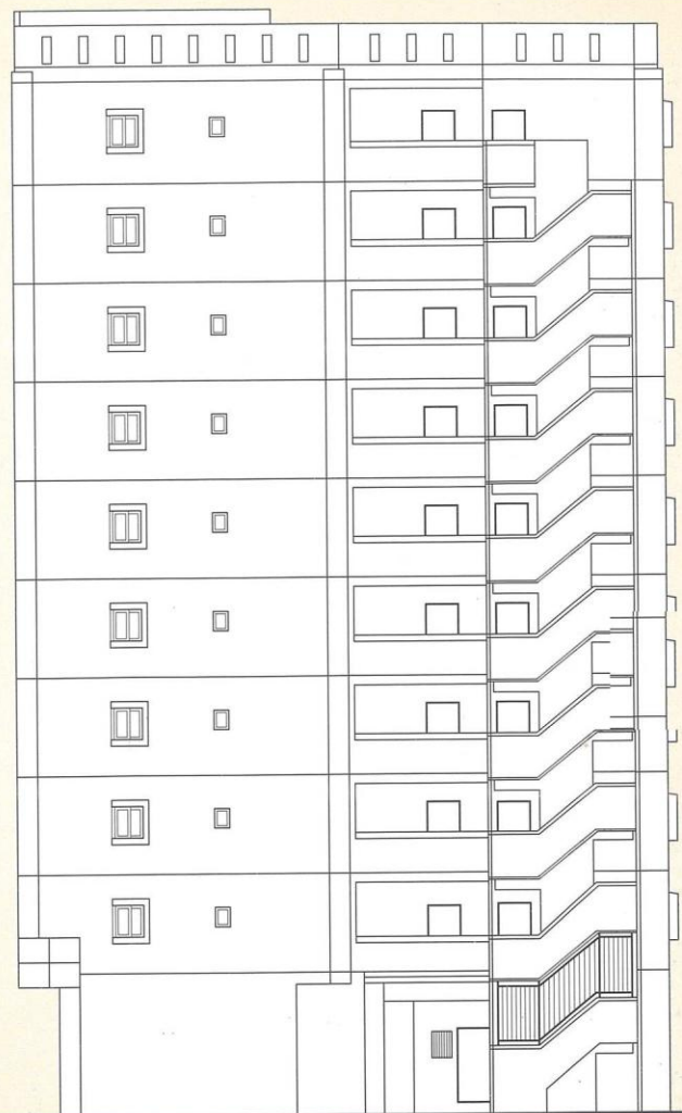
北側立面図
