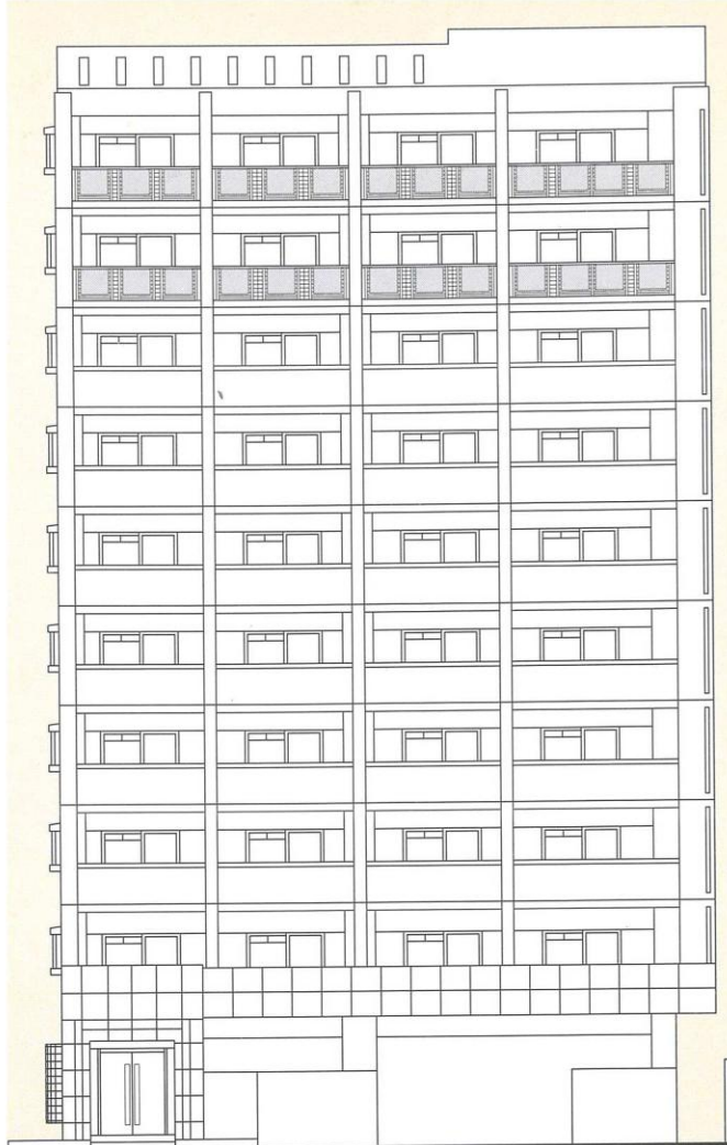
南側立面図
