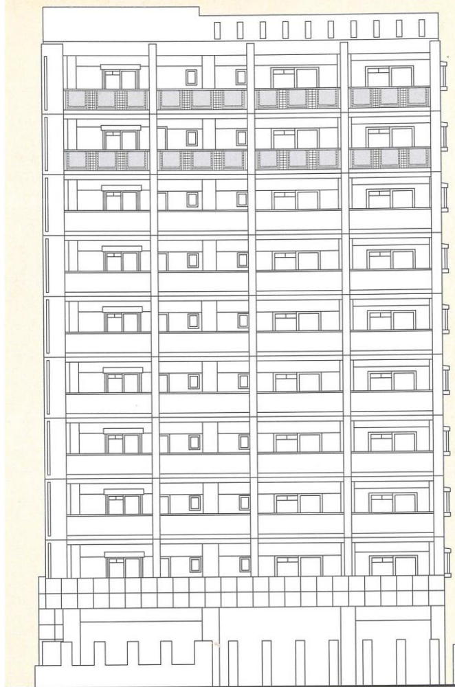
東側立面図
