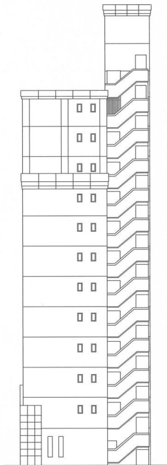
西側立面図
