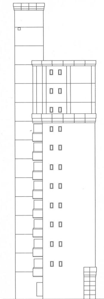
東側立面図
