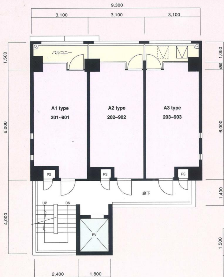
2～9階平面図
