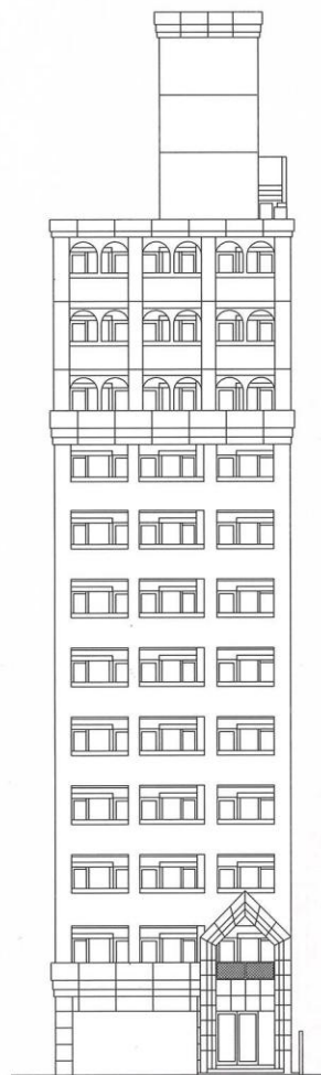
北側立面図
