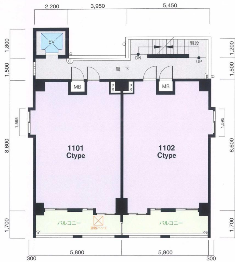
11階平面図
