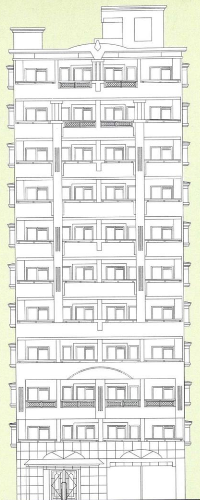
南側立面図
