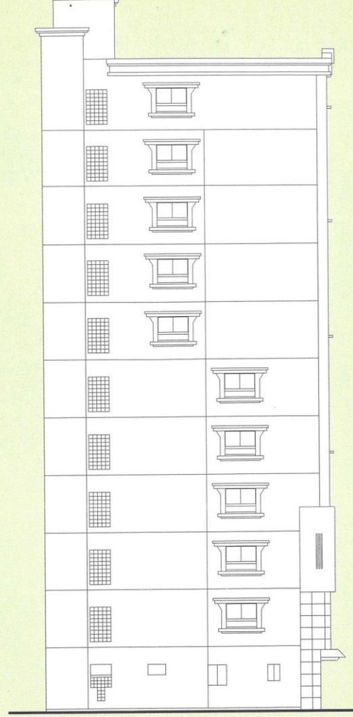
西側立面図
