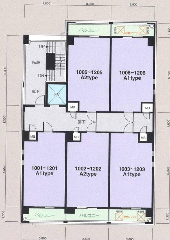
10~12階平面図
