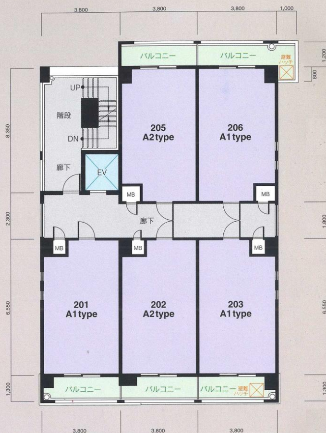
2階平面図
