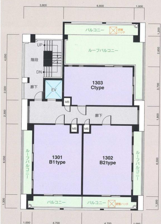
13階平面図
