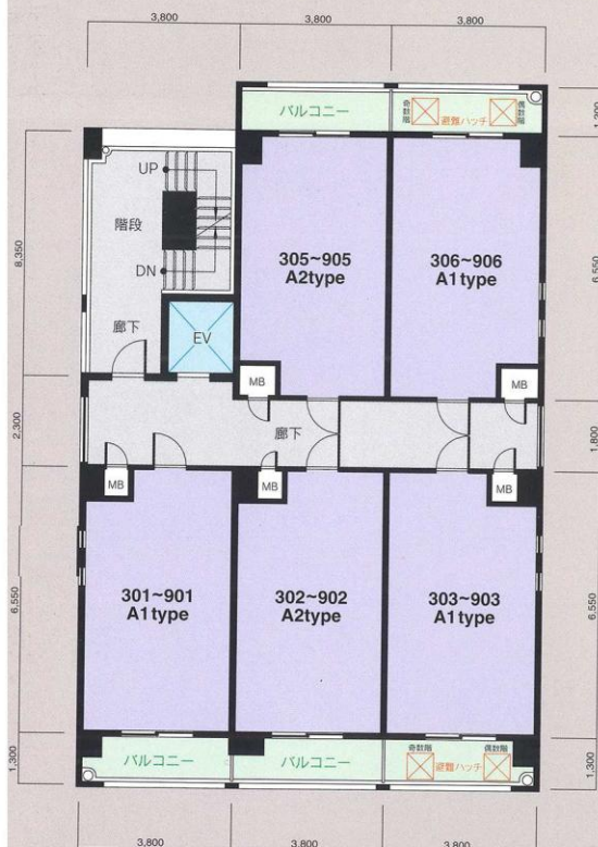
3~9階平面図
