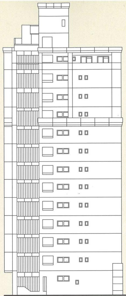
西側立面図
