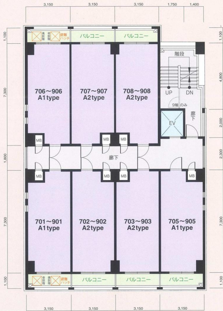
7～9階平面図
