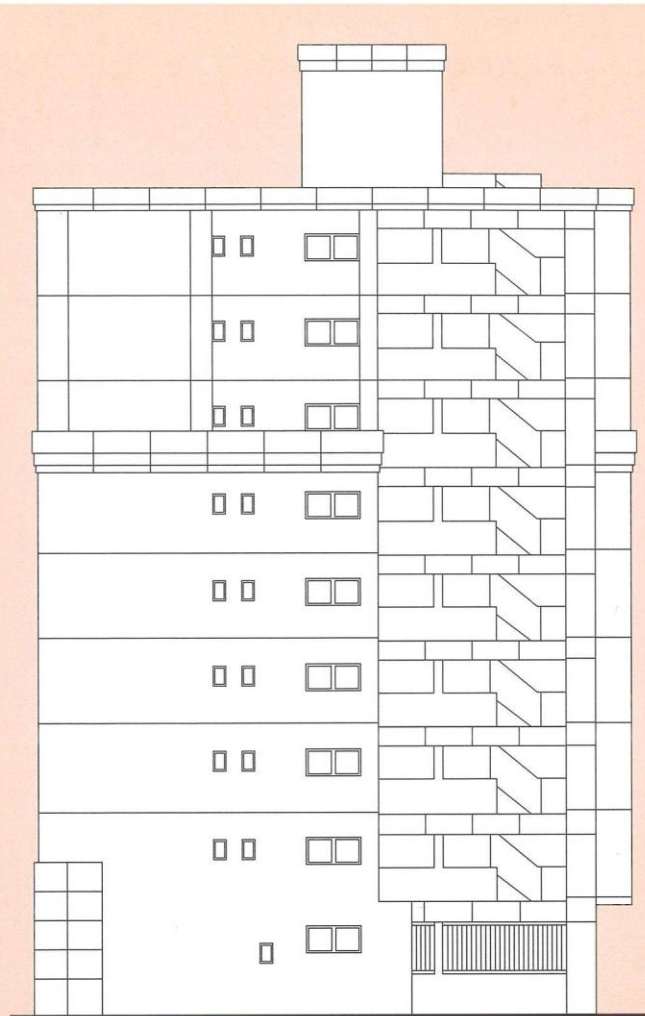
東側立面図
