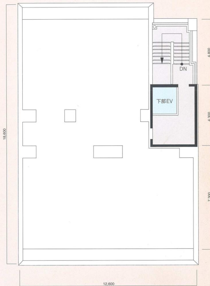
RH階平面図
