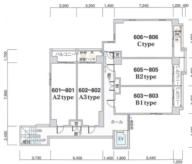
6~8階 平面図
