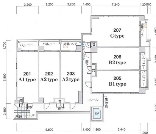
2階 平面図
