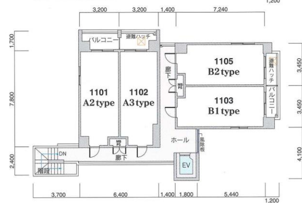
11階 平面図
