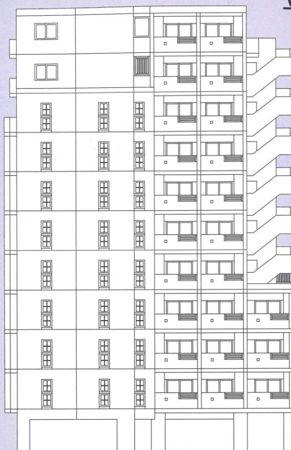
东侧立面图
