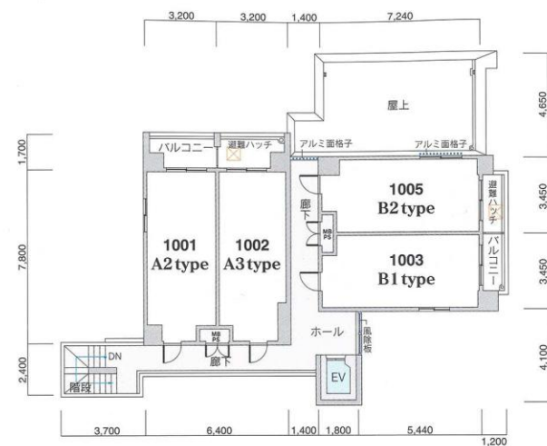
10階 平面図
