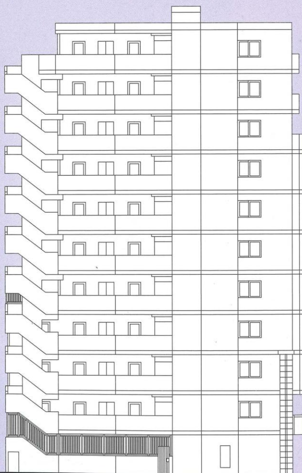
西侧立面图
