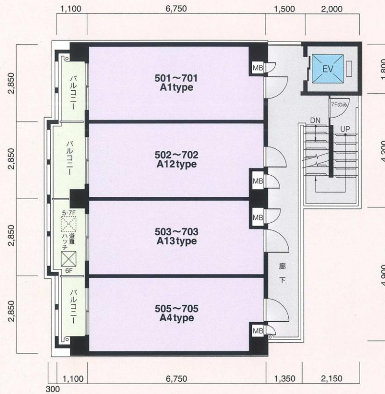
5~7F平面図
