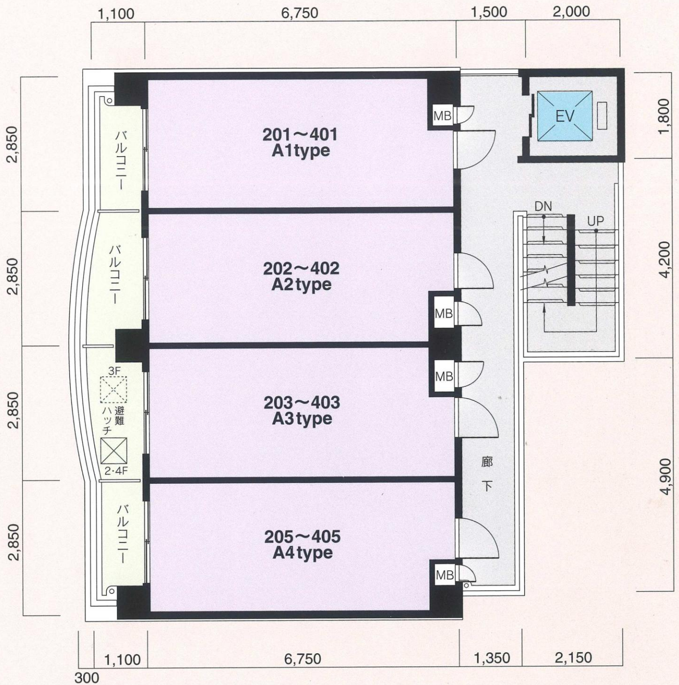
2～4F平面図
