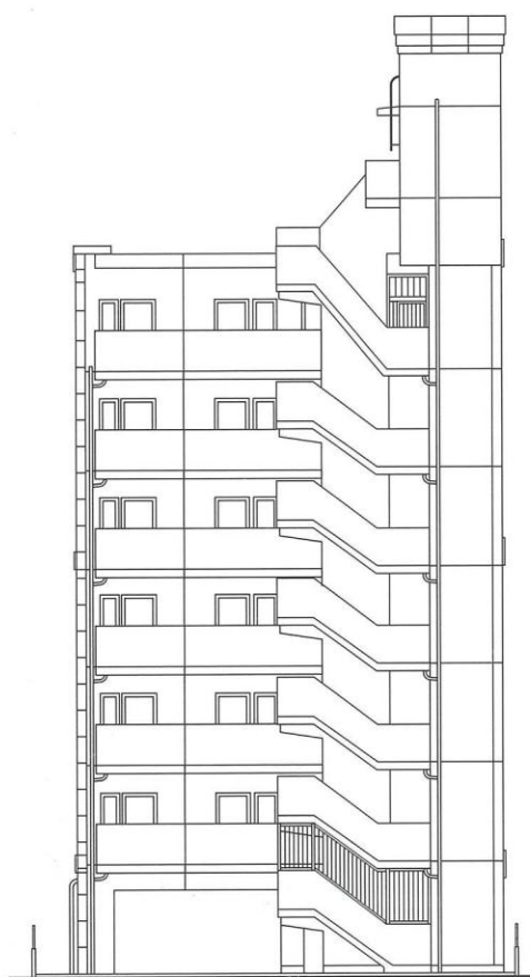
南側立面图
