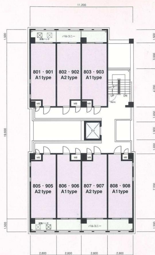
8・9階平面図
