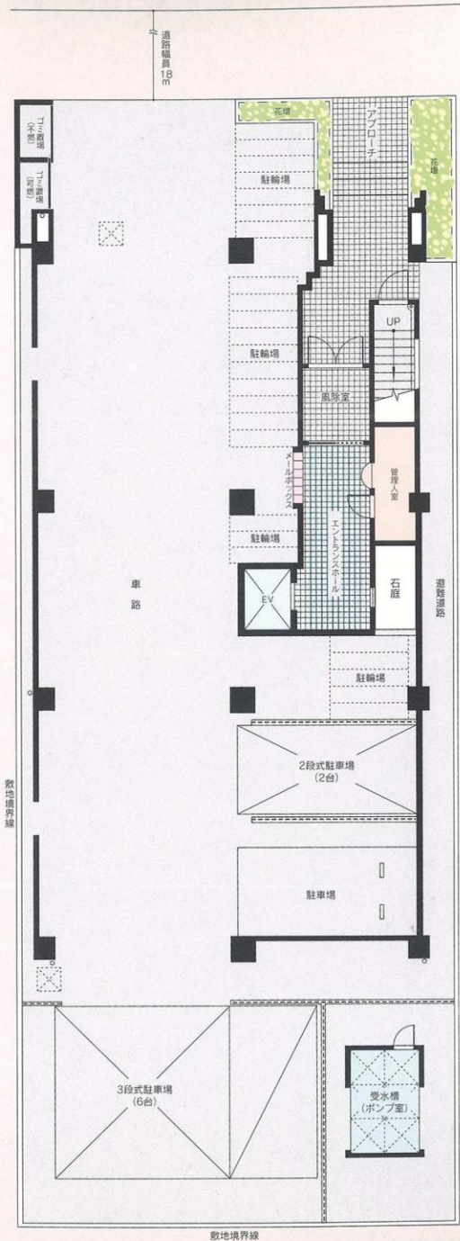
配置図・1階平面図
