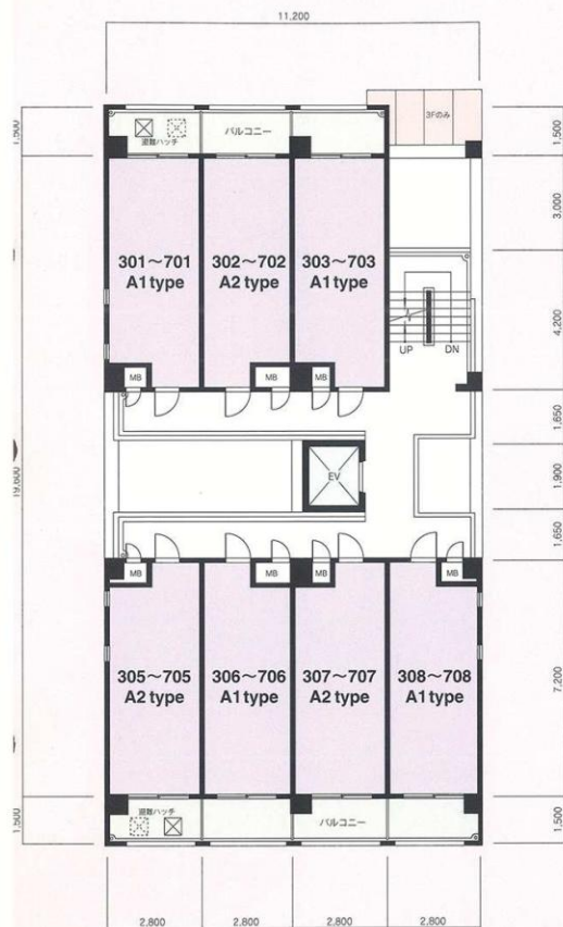
3~7階平面図
