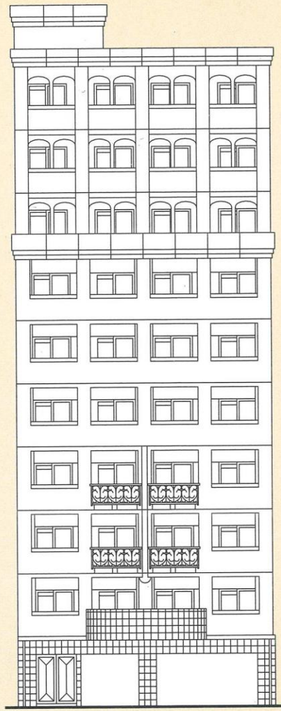
北側立面図
